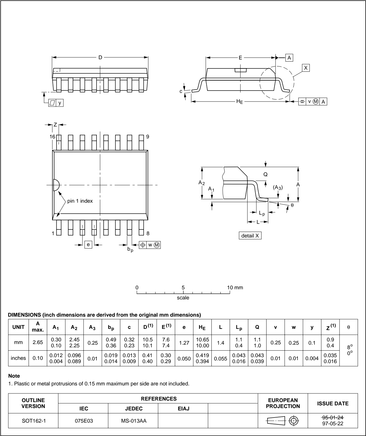
Fig 17. SOT162-1.
