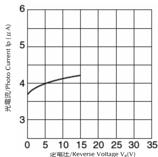
逆電圧—光電流 特性
