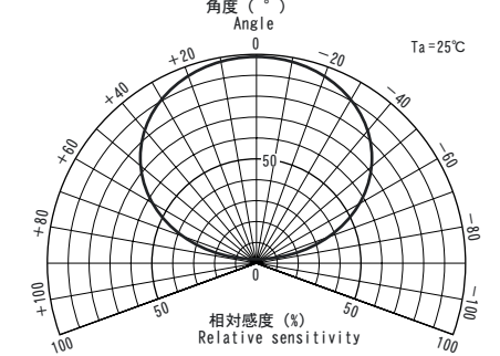
■指向特性
