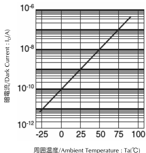
周囲温度—暗電流 特性 Ambient Temperature vs. Dark Current 条件/Condition : V_R = 10\text{V}
