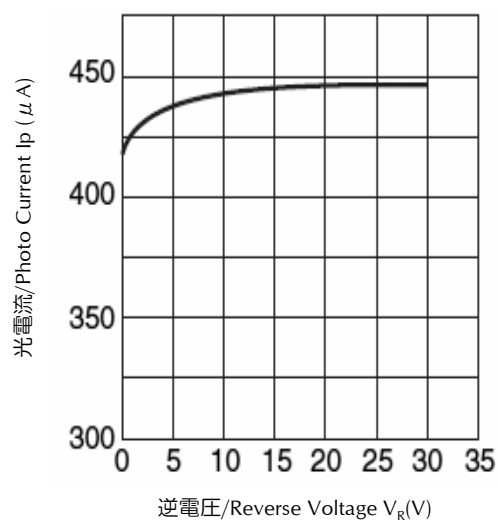
逆電圧—光電流 特性
