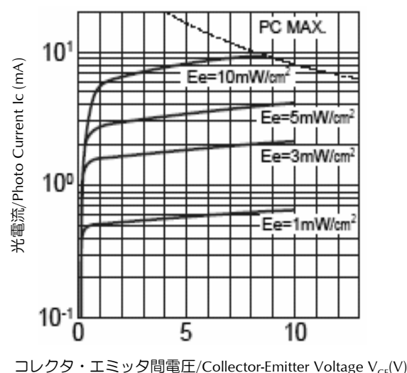
コレクタ・エミッタ間電圧—光電流 特性 Collector-Emitter Voltage vs. Photo Current 条件/Condition : T_a = 25^\circ\text{C}
