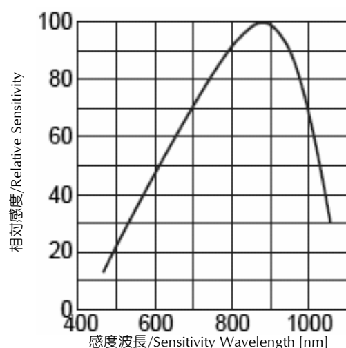
スペクトル分布特性 Relative Sensitivity vs. Sensitivity Wavelength 条件/Condition : T_a = 25^\circ\text{C} , V_{CE} = 5\text{V}
