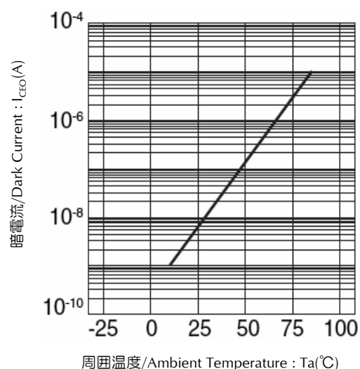
周囲温度—暗電流 特性 Ambient Temperature vs. Dark Current
