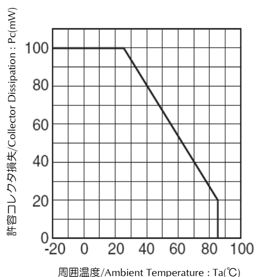
コレクタ損失低減曲線 Ambient Temperature vs. Collector Dissipation
