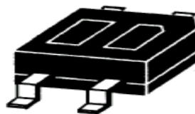
フォトリフレクタ CNB1001 CNB1002 CNB2001 CNB1011
