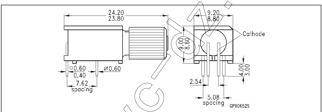
SFH 752V
