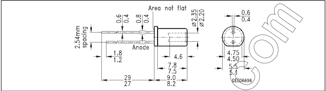
SFH 752
