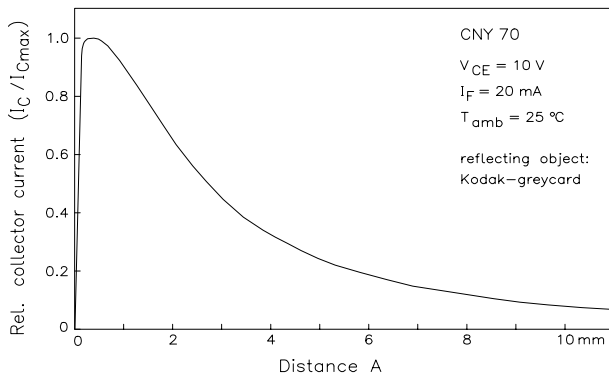
b) CNY 70
