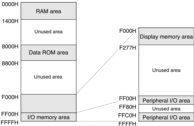
Fig. 4.1.1 Memory map
