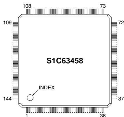
QFP8-144pin
