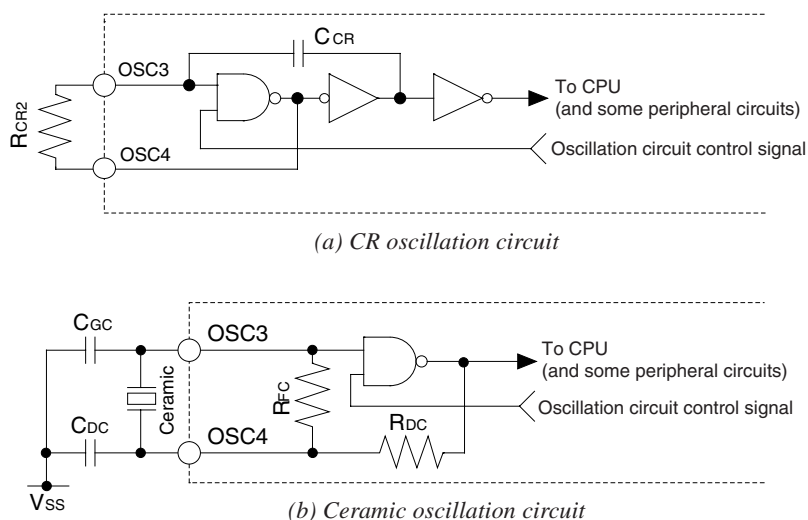
Fig. 4.3.3.1 OSC3 oscillation circuit
