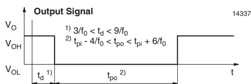
Fig. 1 - Output Function
