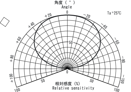
■ 指向特性
