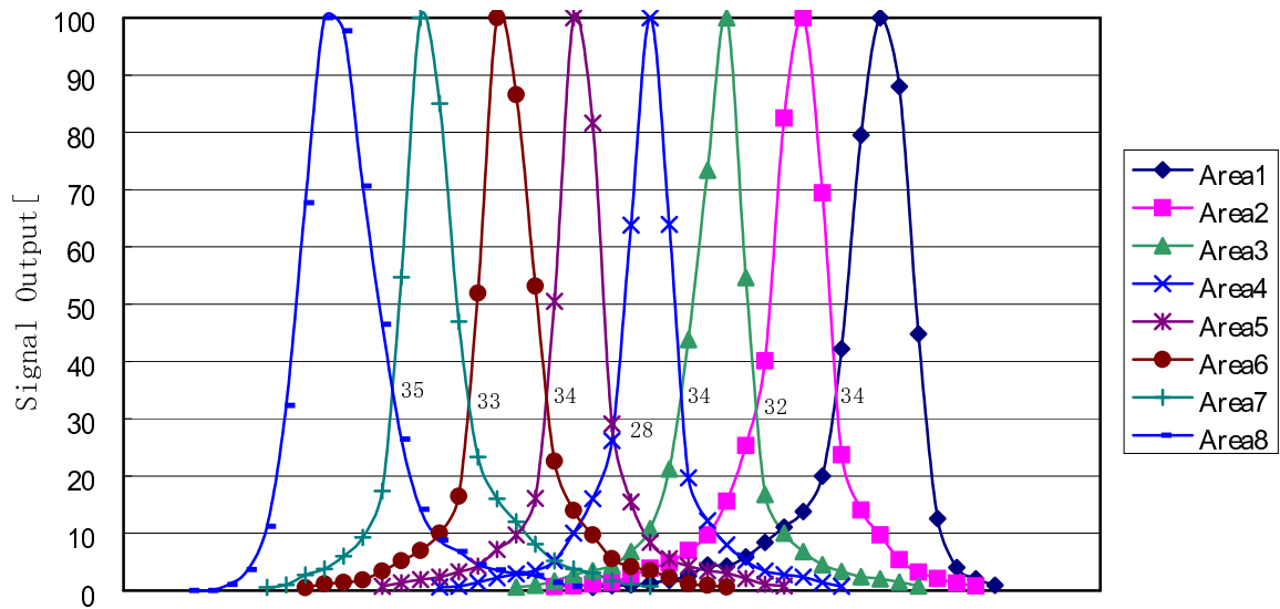
Fig. 4 : Crosstalk (Typ. Value)
