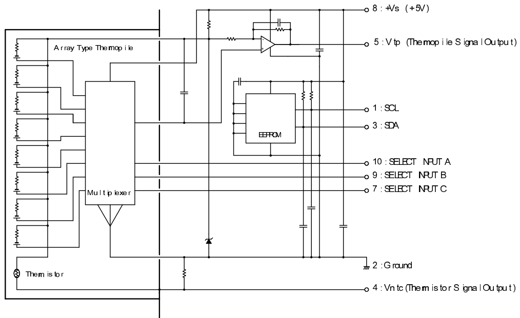
Fig. 2 : Circuit Configuration
