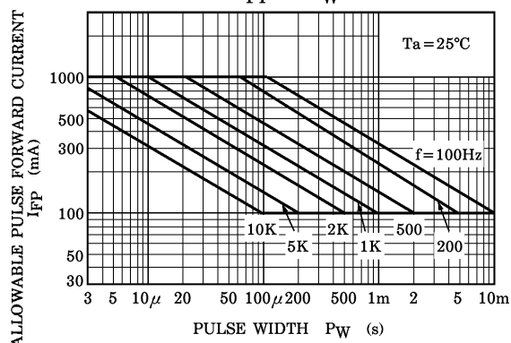
I_{FP} - P_W
