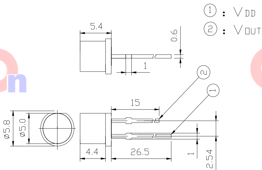
Fig. 14 普通 \Phi 5\text{mm} 平头直插型外形封装尺寸
