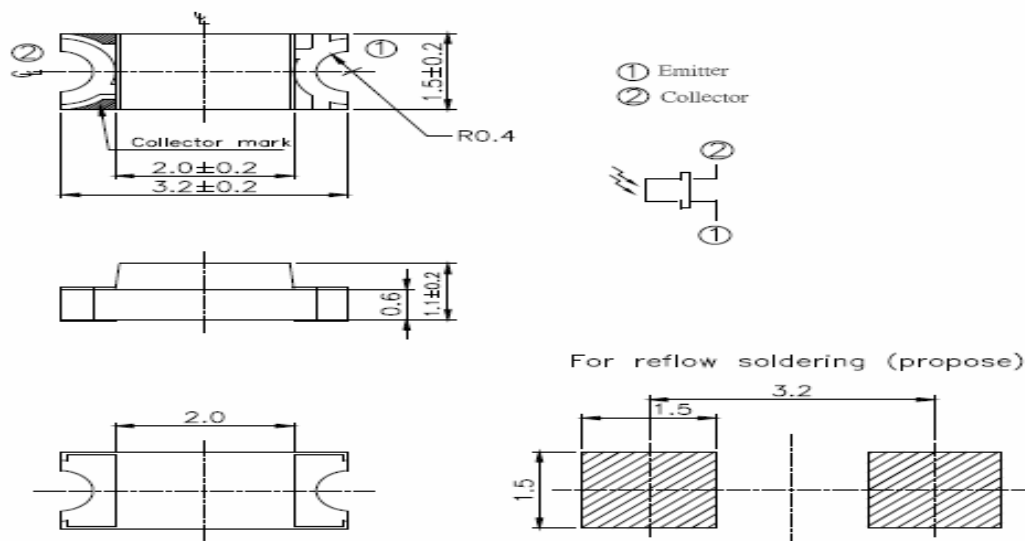
Fig. 15 普通1206 贴片型外形封装尺寸
