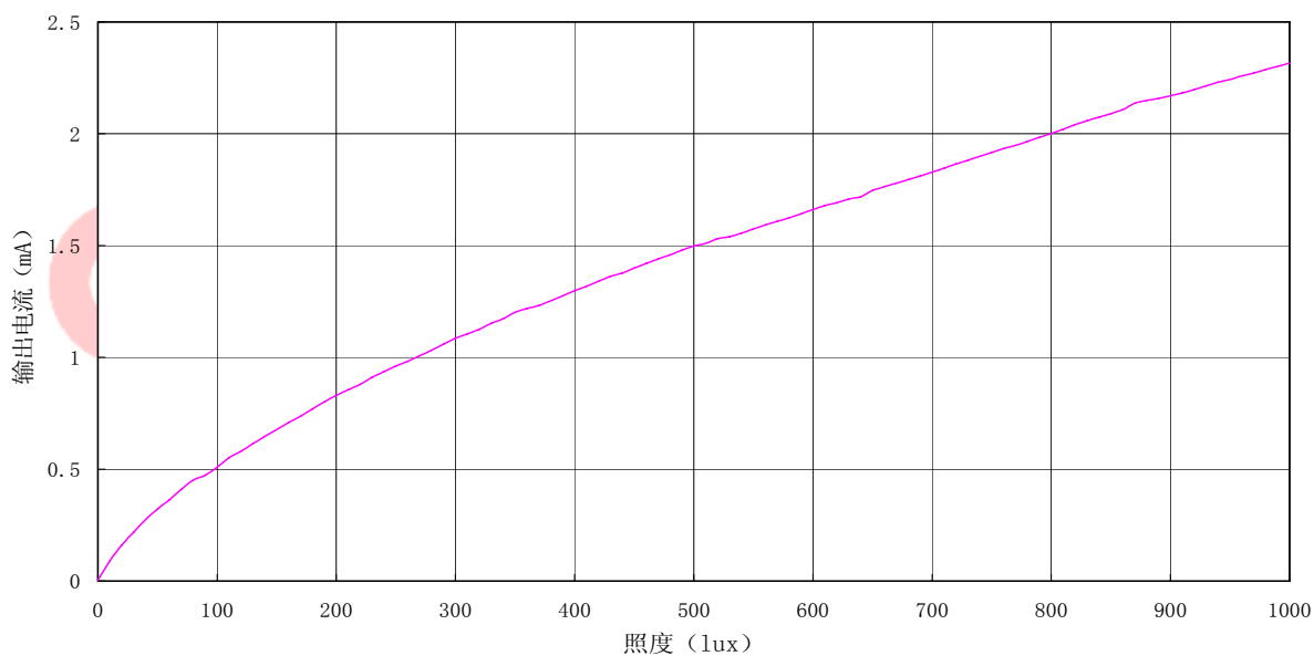
Fig. 6 白炽灯光照响应输出电流曲线
