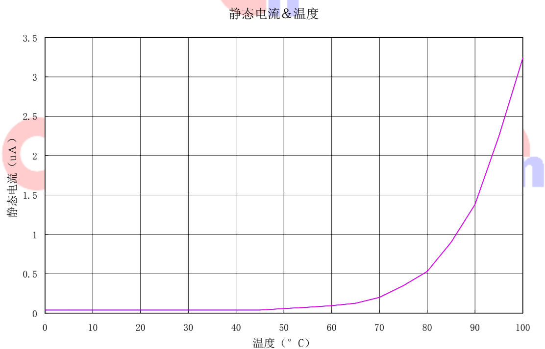
Fig.8 静态电流随温度变化的曲线
