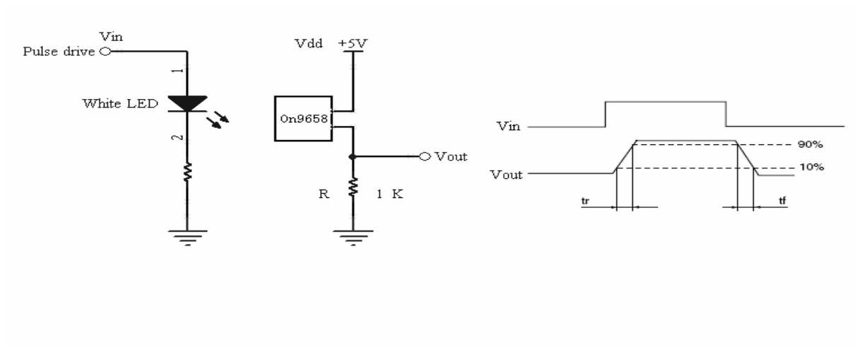
Fig. 5 开光时间测试电路
