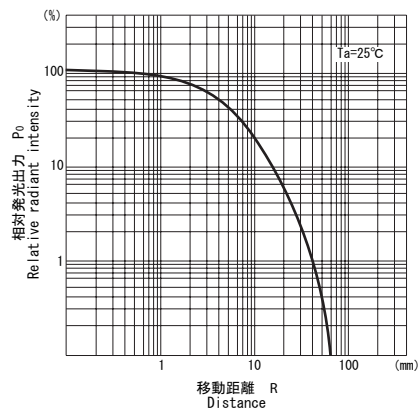
■相対発光出力／距離特性 P_0/R^{\ast 1}
