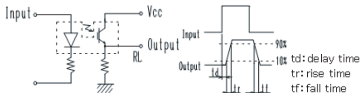
*1 応答時間特性
