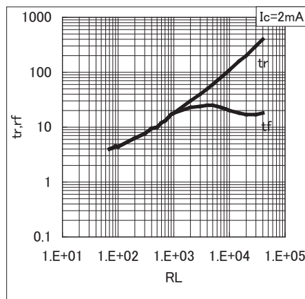
*1 応答時間特性図
