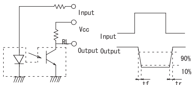
*1 応答時間特性図
