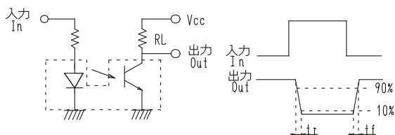
*1応答時間測定回路
