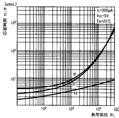
■応答時間/負荷抵抗特性 t_r, t_f/R_L *
