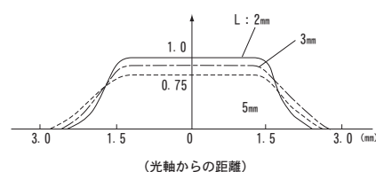
■相対光強度分布 ※2 RADIATION PATTERN
