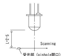
※2 相対光強度分布 測定方法
