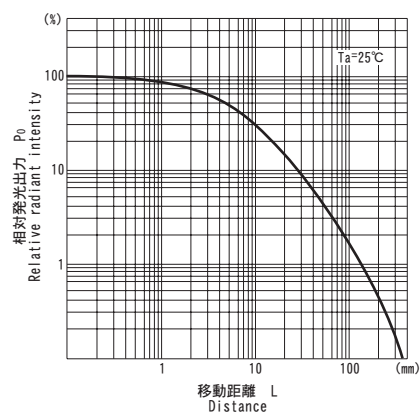
■相対発光出力／距離特性 P_0/L
