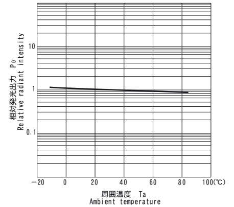
■相対発光出力／周囲温度特性 P_O/T_a
