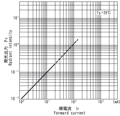
■発光出力／順電流特性 P_O/I_F (mW)
