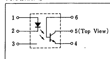
内部接続図/Pin Connection
